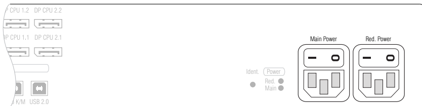
Abbildung 5: Schnittstellen zum Anschluss der Stromversorgung
